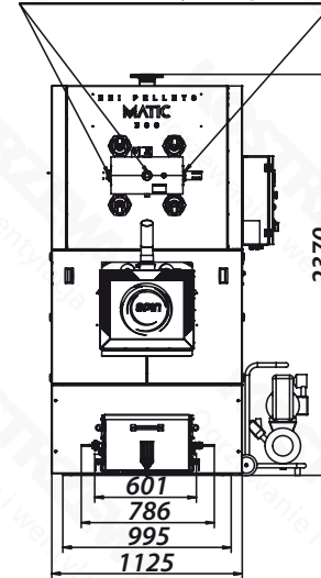
Króćce 1 1/2" czyszczenia pneumatycznego
