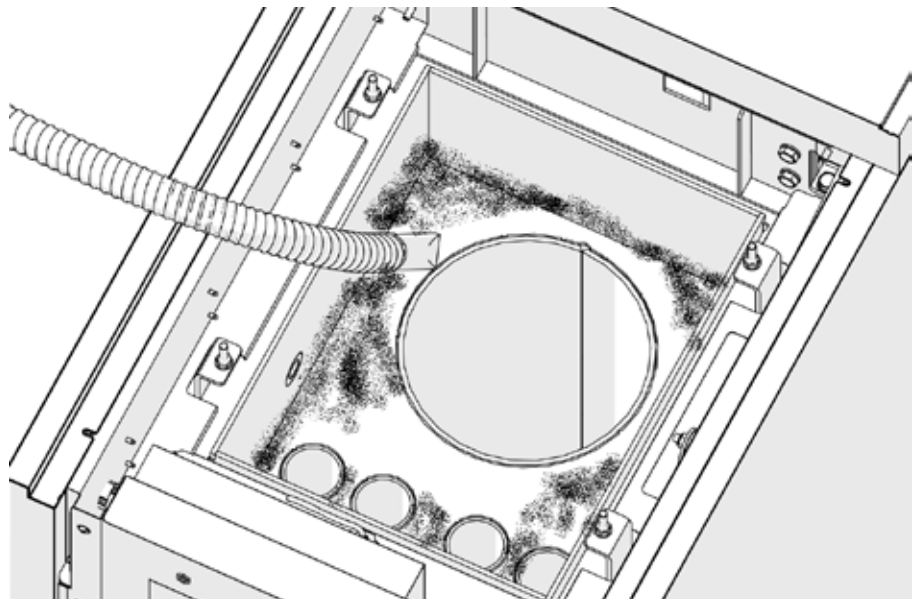
Rys. Czyszczenie pozostałości popiołu w górnej części wymiennika
