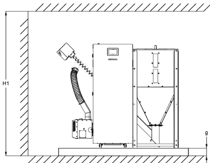
Rys: Schemat wymiarowy (na górze - widok z boku, na dole od lewej: widok z przodu, widok z tyłu).
