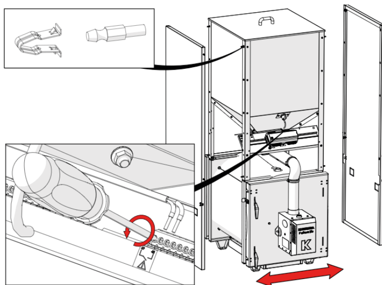
Rys: Montaż / demontaż czujnika otwarcia drzwiczek
