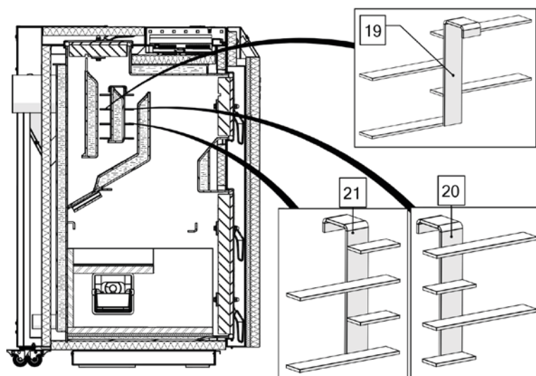
Rys.: Zestaw zawieszający oraz ich umiejscowienie w kotle Twin Bio Luxury Compact typ NE 8-12
