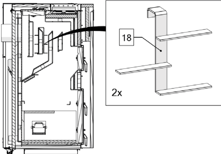
Rys: Rysunek 4. Zestaw zawieszający oraz ich umiejscowienie w kotle Twin Bio Luxury Compact typ NE 16 – 24
