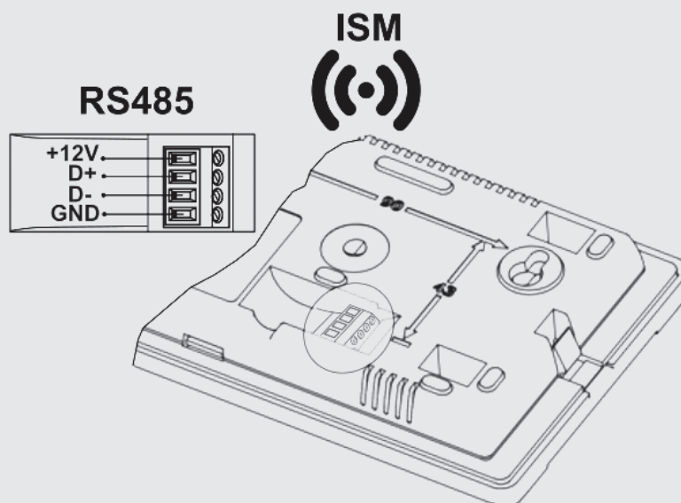
Panel pokojowy ecoSTER TOUCH_K30 bezprzewodowy
