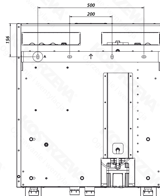
ROZSTAW OTWORÓW MONTAŻOWYCH
