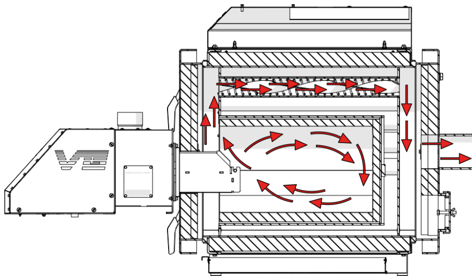
Rysunek 6.2. Obieg spalin w kotle Mini Bio Luxury B.
