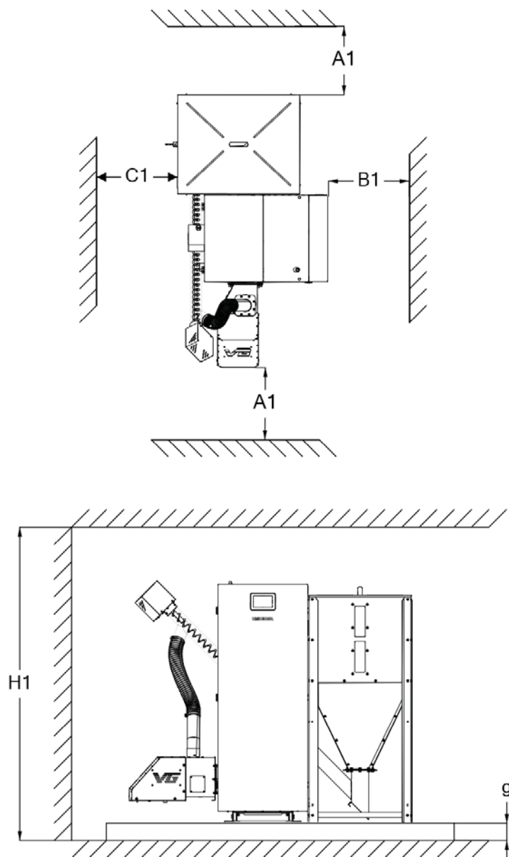
Rys: Schemat wymiarowy (na górze - widok z boku, na dole od lewej: widok z przodu, widok z tyłu).
