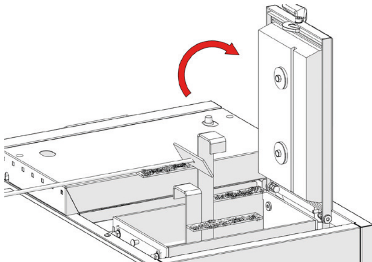
Rys: Zawirowywacz dla mocy 16, 24kW
