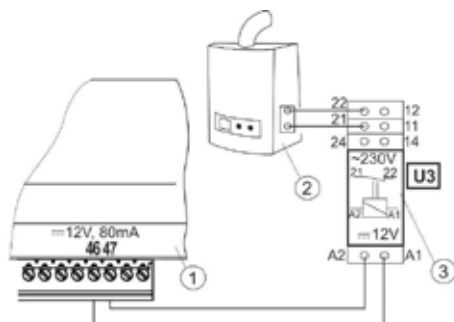
Przykładowy schemat układu do podłączenia kotła rezerwowego do regulatora:
